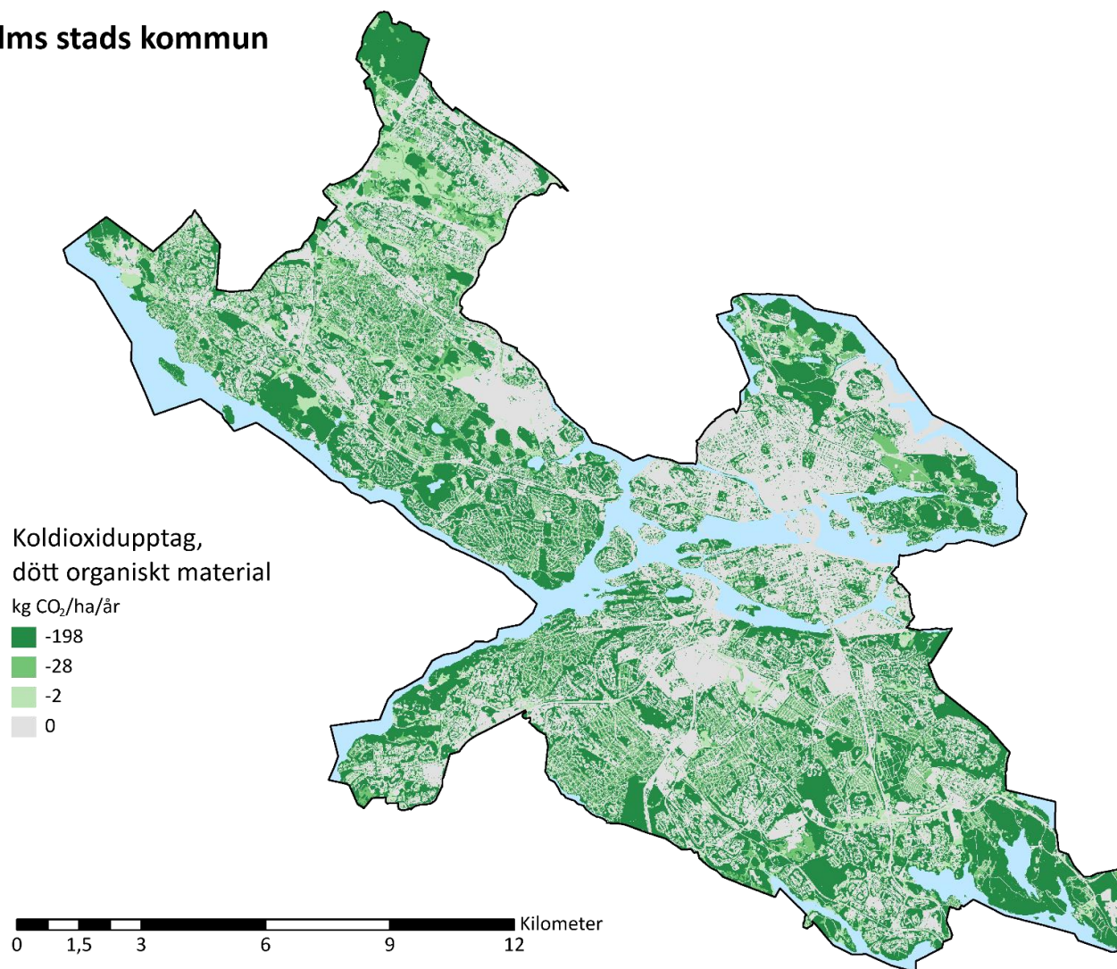
Figur 15. Totalt koldioxidupptag av dött organiskt material på marker, inom Stockholms stad.
