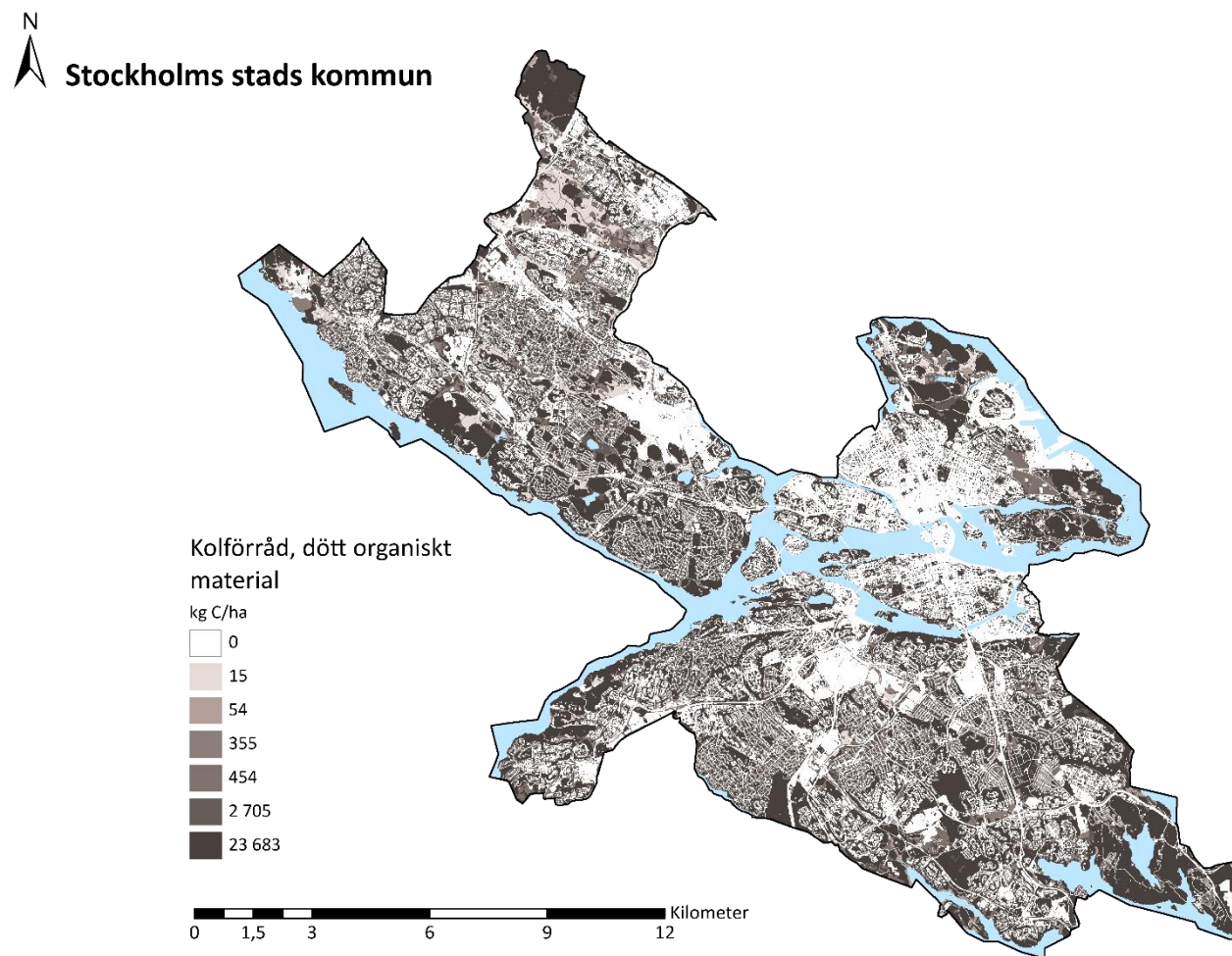
Figur 9. Totalt kolförråd i dött organiskt material på marker inom Stockholms stad.
