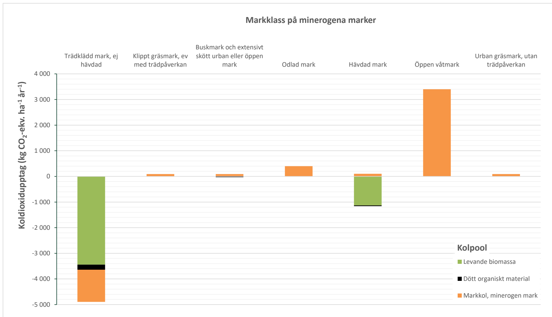
Figur 11. Genomsnittligt koldioxidupptag per ytenhet av minerogen mark i Stockholms stad fördelat på markklasser och kolpooler. Markklasser med försumbart koldioxidupptag visas ej.
