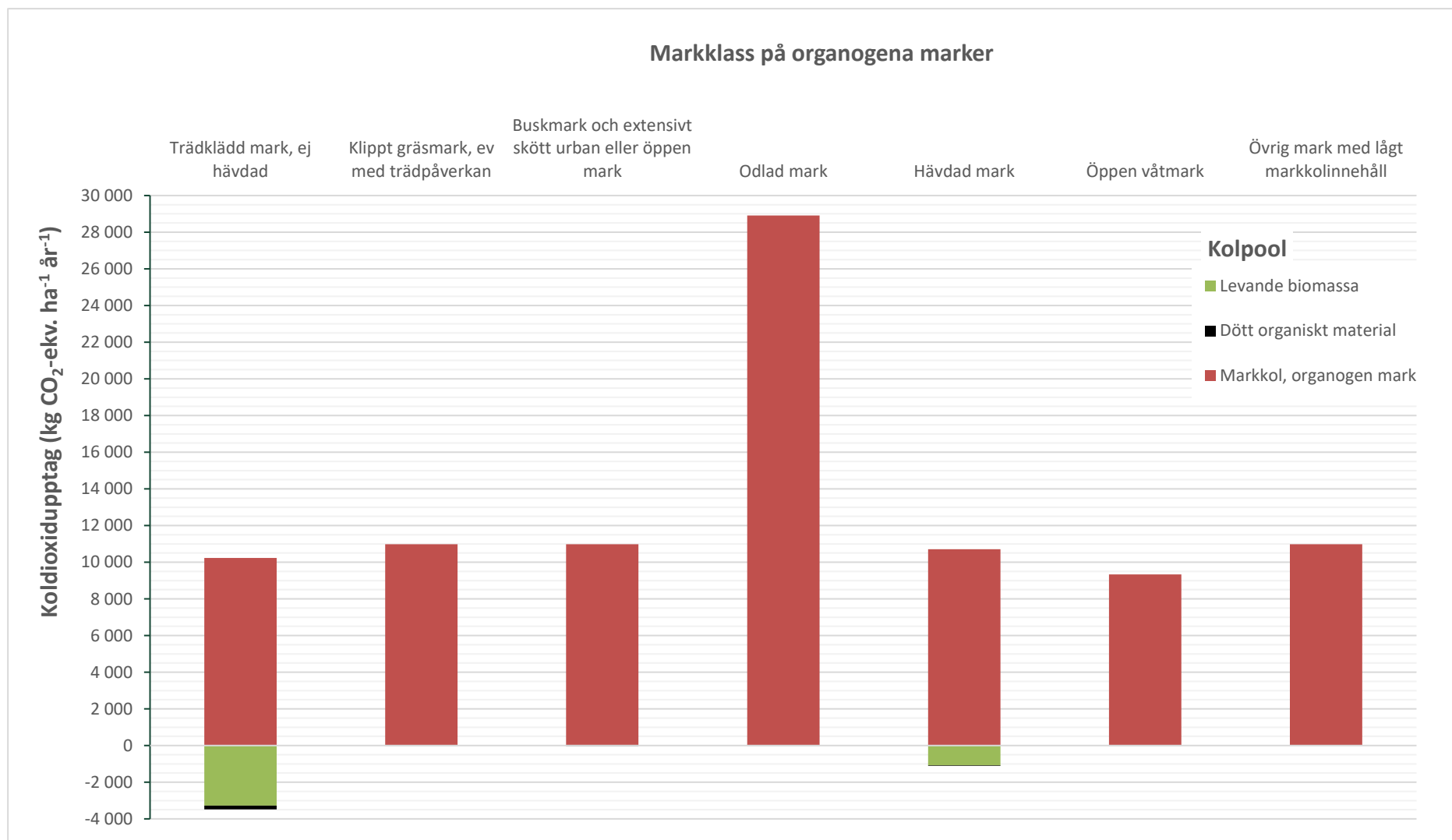
Figur 12. Genomsnittligt koldioxidupptag per ytenhet av organogen mark i Stockholms stad fördelat på markklasser och kolpooler. Markklasser med försumbart koldioxidupptag visas ej.
