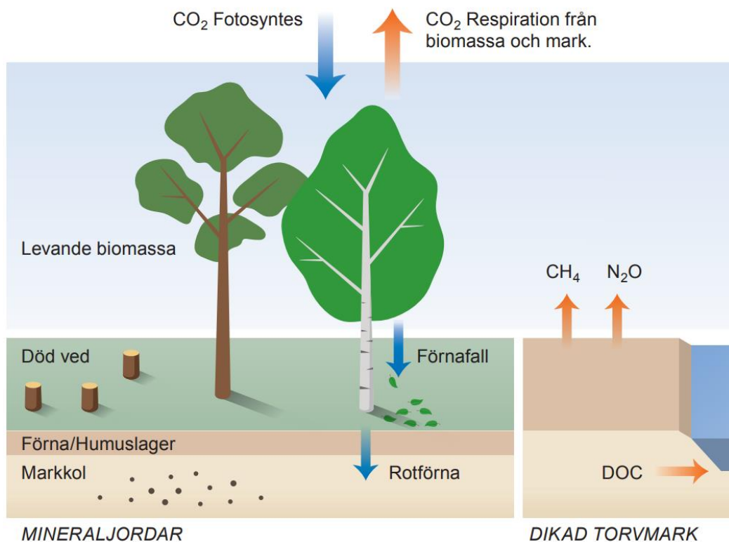
Figur 1. Kolets kretslopp inom kolpoolerna i skog och mark.
