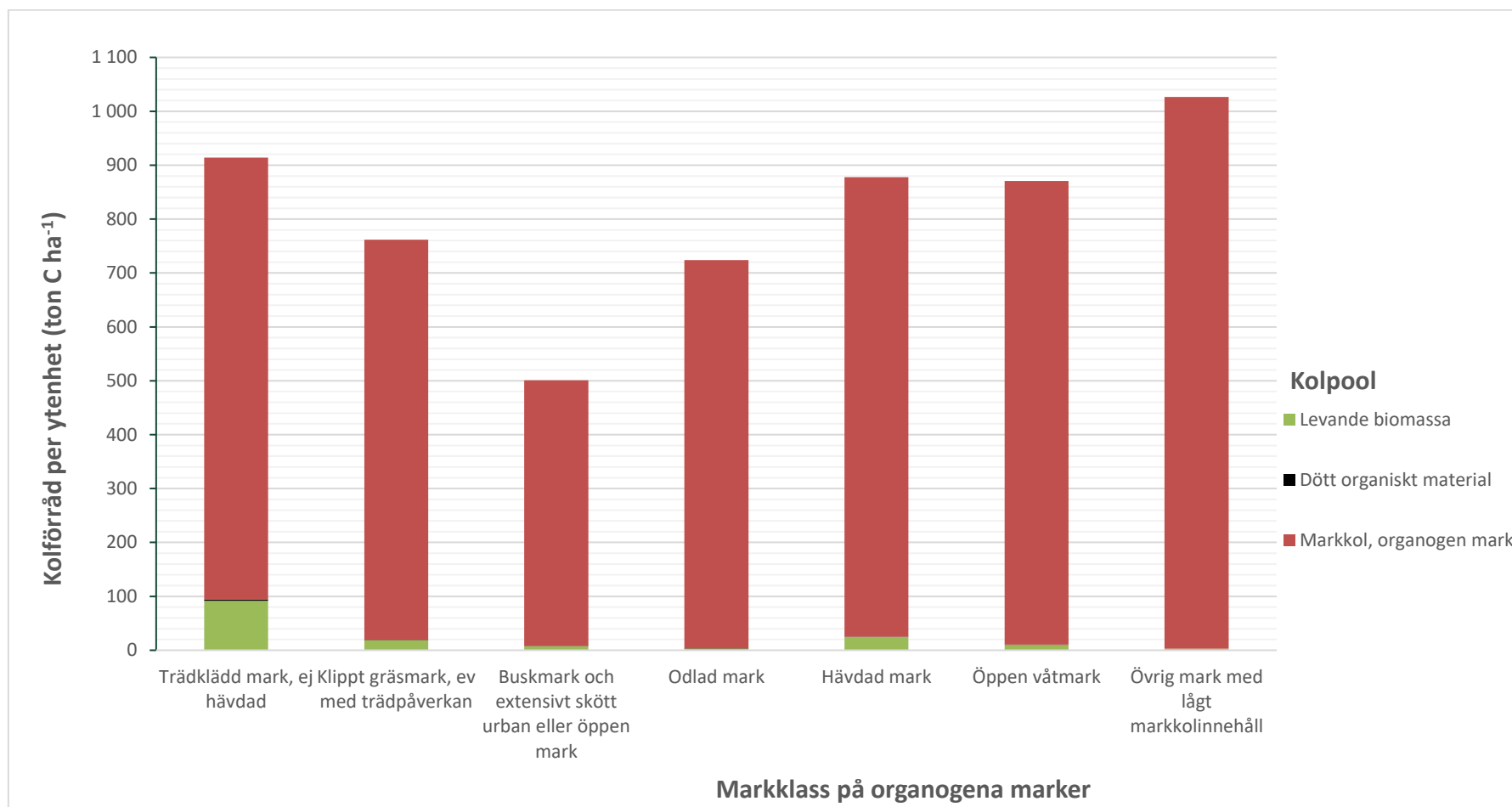
Figur 6. Genomsnittligt kolförråd per ytenhet för organogen mark inom Stockholms stad fördelat på markklasser och kolpooler. Markklasser med försumbart kolförråd visas ej.
