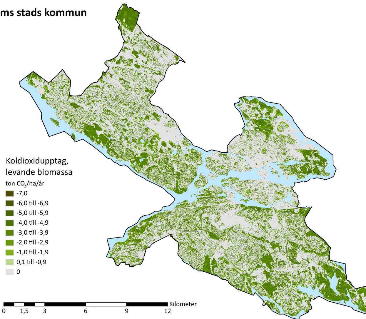
Figur 14. Koldioxidupptag av levande trädbiomassa, inom Stockholms stad.
