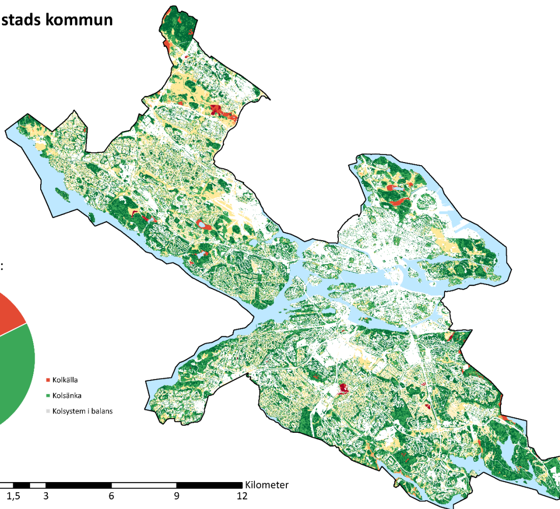
Figur 13. Totalt koldioxidupptag av skog och mark, inom Stockholms stad.
