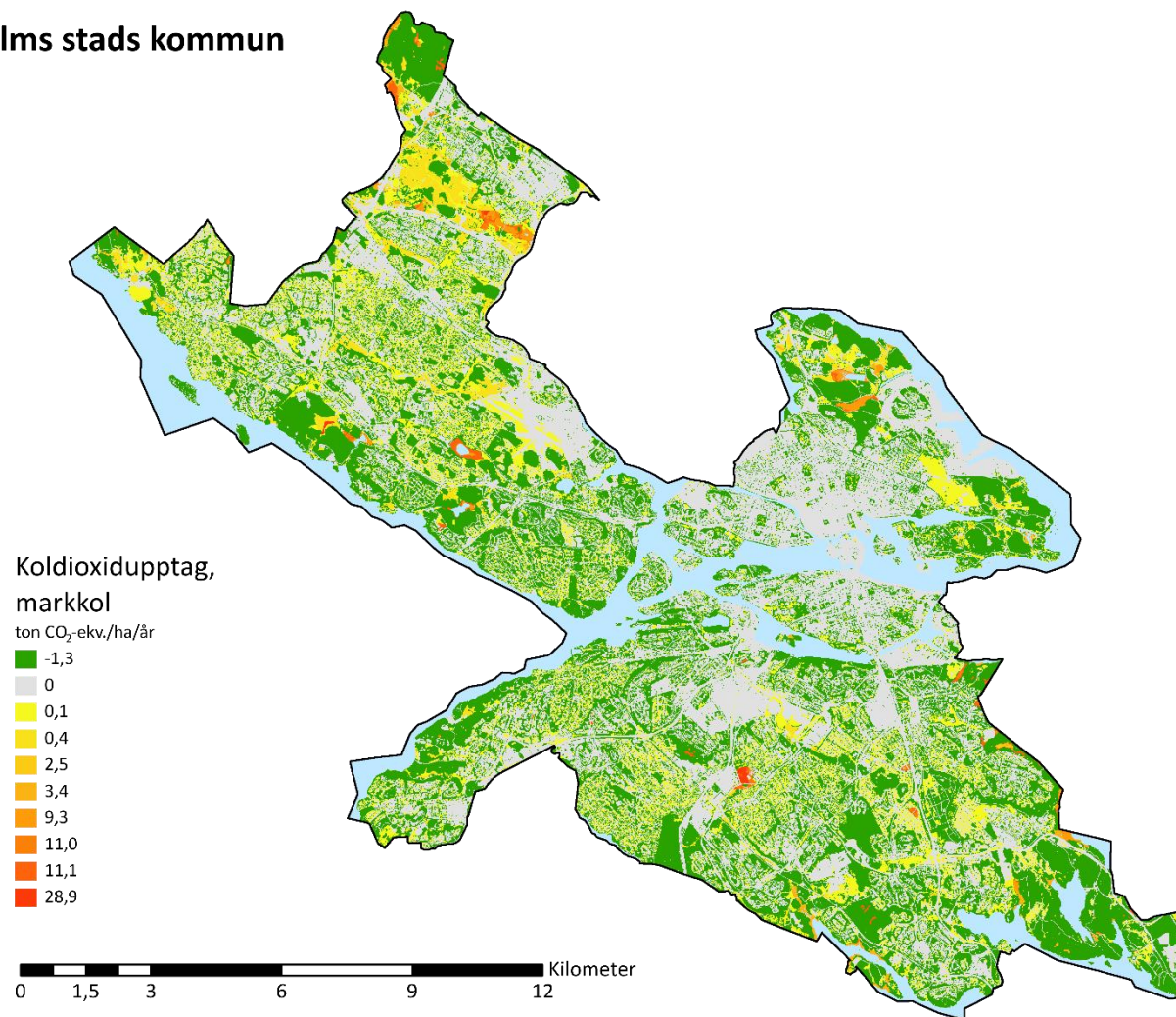
Figur 16. Totalt koldioxidupptag av markkol, inom Stockholms stad.
