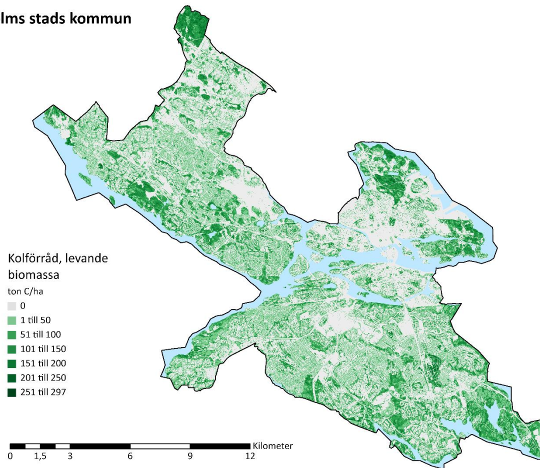
Figur 8. Kolförråd i levande trädbiomassa inom Stockholms stad.
