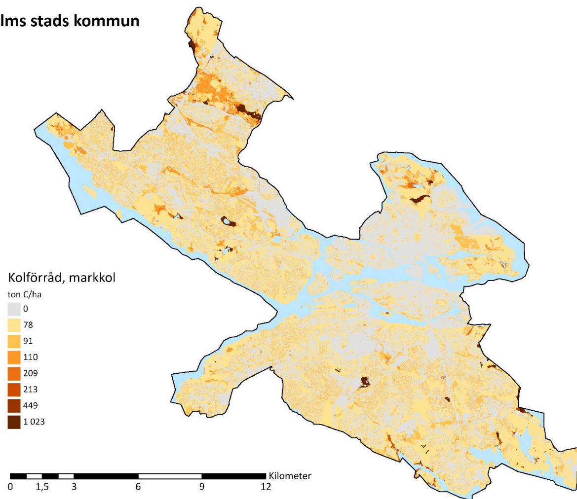
Figur 10. Markkolets kolförråd inom Stockholms stad.
