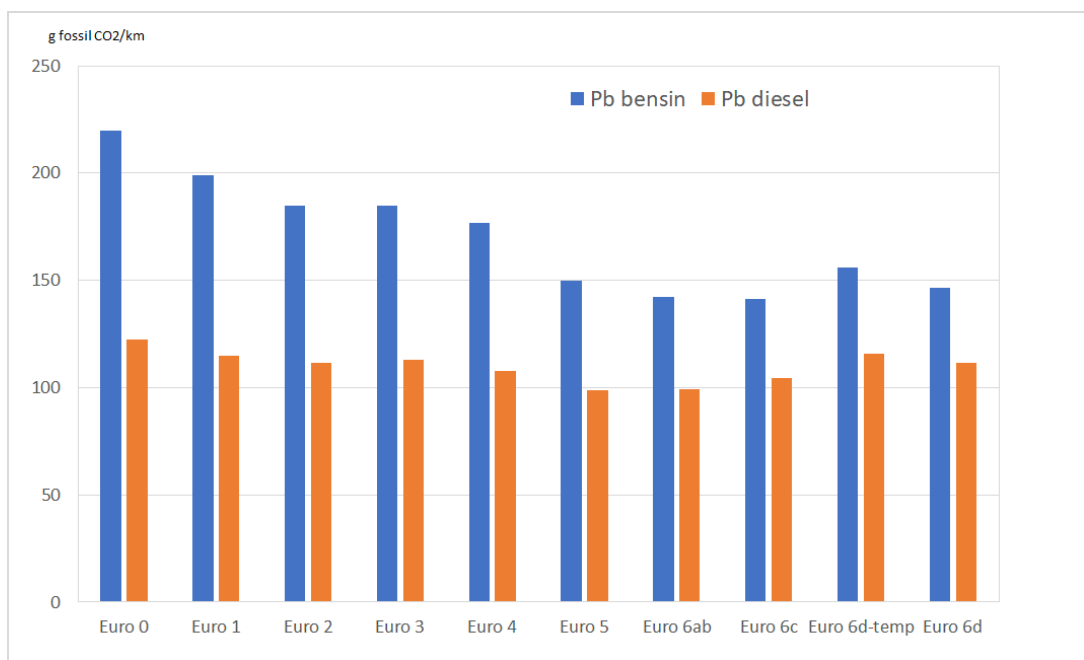
Figur 14. Utsläpp av koldioxid, \text{CO}_2 , g/km för personbilar, bensin resp. diesel, uppdelat på olika euroklasser för Hornsgatans vägtyp. HBEFA 4.1 [7] med avräkning av 6 % inblandning av biodrivmedel i bensin och 37 % i diesel, se Bilaga 4.
