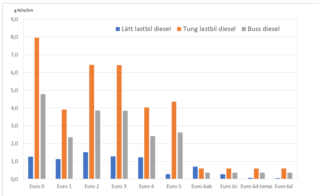
Figur 13. Utsläpp av kväveoxider, \text{NO}_x , g/km för lätta- och tunga diesellastbilar samt tunga dieselbussar uppdelat på olika euroklasser för Hornsgatan. HBEFA 4.1 [7].
