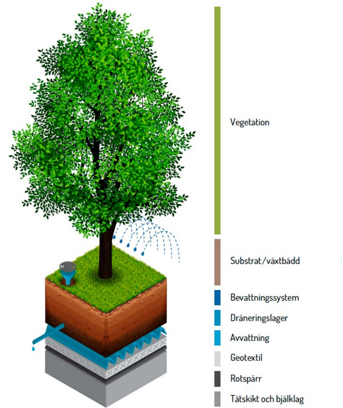
Genomskärning av grönt tak med olika lager ur Grönatakhåndboken www.gronatakhåndboken.se . Illustration: Patrik Granqvist
