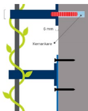
Växtvajer på en befintlig skärm från Urban green
