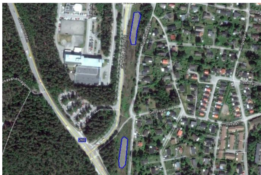
Figur 20. Illustration av ytbehov och ungefärlig placering av två alternativa dagvattendammar vid Skrubba Malmväg på 0,13 hektar (våtyta) vardera, vilket motsvarar cirka 1 % av tillrinningsområdets reducerade yta.
