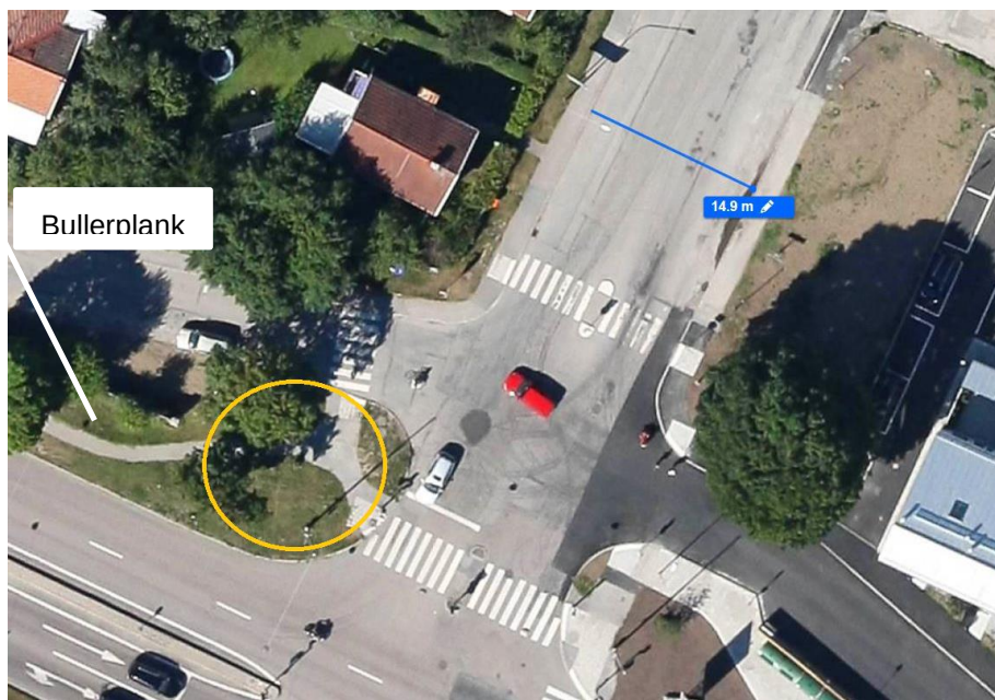
Figur 20 - Korsningen där Vultejustvägen (norrifrån) möter Bergslagsvägen. Mer än halva vägsträckan är ca 15 m lång. Gul cirkel indikerar plats dit vägdagvattnet kan ledas och tas omhand i en växtbädd/regnträdgård.
