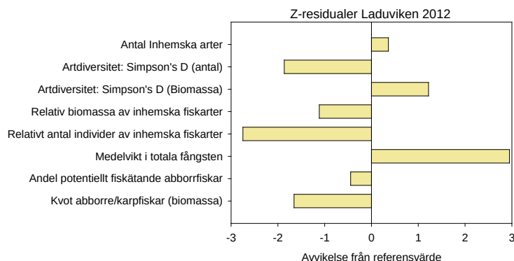
Fig. 11. Z-värden från provfisket i Laduviken. Z-värdena visar om avvikelsen för respektive indikator är högre (större än 0) eller lägre än referensvärdet (mindre än 0). Om Z-värdet är noll överensstämmer provfiskeresultatet med referensvärdet. Medelvikt i totala fångsten samt det relativt antal individer av inhemska arter avvek signifikant.
