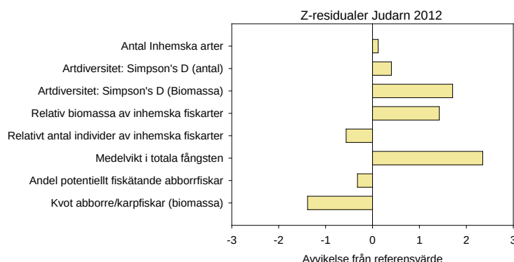
Fig. 5. Z-värden från provfisket i Judarn. Z-värdena visar om avvikelsen för respektive indikator är högre (större än 0) eller lägre än referensvärdet (mindre än 0). Om Z-värdet är noll överensstämmer provfiskeresultatet med referensvärdet. Medelvikten i totala fångsten avvek signifikant.
