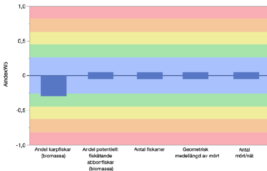
Figur 48. Den ekologiska statusen uppdelat på de fem parametrarna i det multimetriska surhetsindexet AindexW5 i Drevviken 2021. Avvikelse från referenstillståndet visas med skala normaliserad till värden mellan -1 och 1 för att utfallet för samtliga parametrar lättare ska kunna utläsas ur samma Figur. Färgerna visar statusklass där blå=hög status, grön=god, gul=måttlig, orange=otillfredsställande och röd=dålig status.
