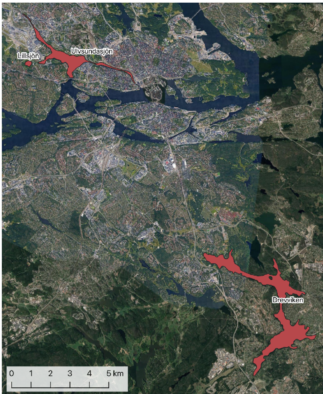
Figur 1. De tre sjöarnas placering (rödmarkerade)
