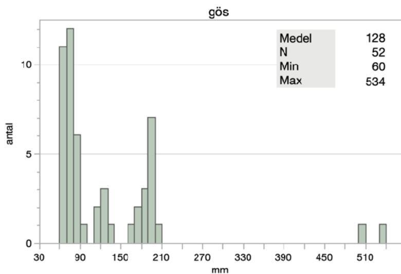
Figur 7. Gösens längdfördelning vid provfisket i Lillsjön 2021.
