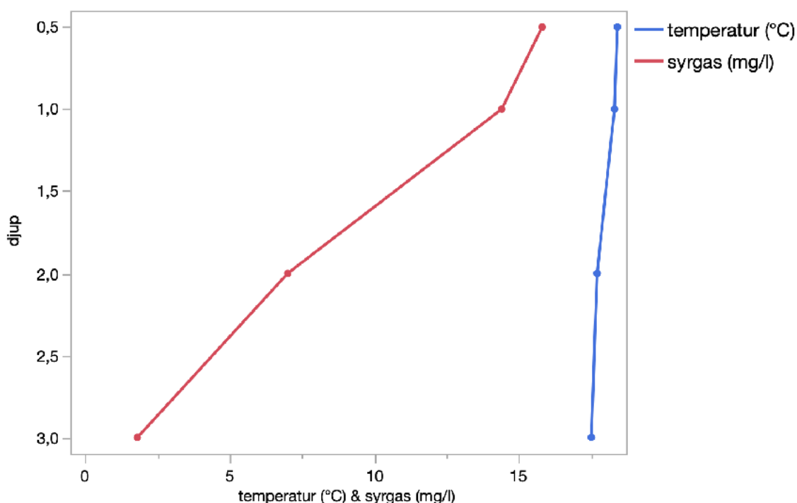
Figur 4. Temperatur- och syrgasprofil i Lillsjön den 23 augusti 2021.
