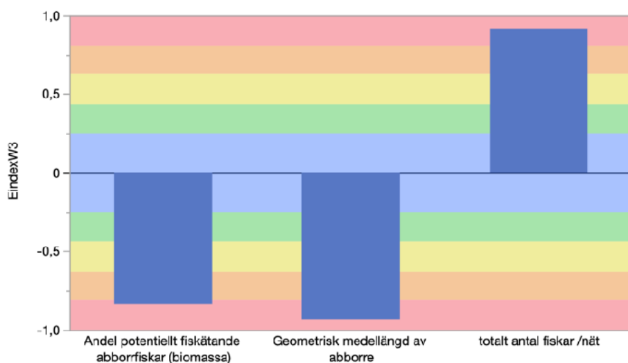
Figur 49. Den ekologiska statusen uppdelat på de tre parametrarna i det multimetriska eutrofiindexet EindexW3 i Drevviken 2021. Avvikelse från referenstillståndet visas med skala normaliserad till värden mellan -1 och 1 för att utfallet för samtliga parametrar lättare ska kunna utläsas ur samma Figur. Färgerna visar statusklass där blå=hög status, grön=god, gul=måttlig, orange=otillfredsställande och röd=dålig status.
