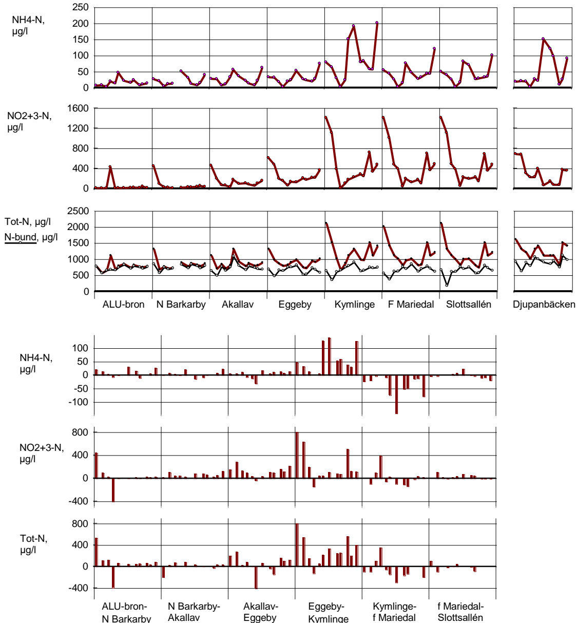
Figur 12. Ammoniumkväve, nitrit+nitratkväve och totalkväve i Igelbäcken och Djupanbäcken januari-december 2014. I diagrammet för totalkväve visas även halterna av bundet kväve. De tre undre diagrammen visar förändringar mellan provpunkterna.
