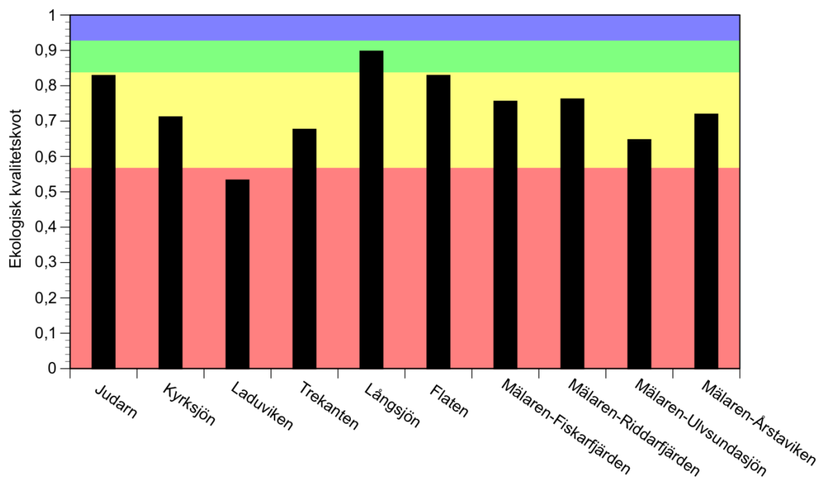
Figur 7. Ekologisk kvalitetskvot för makrofytter i de sex sjöarna och fyra mälarfjärdarna baserat på data från inventeringen 2014. Färgerna motsvarar intervall för respektive statusklass (blå – hög, grön – god, gul – måttlig, röd – otillfredsställande/dålig).
