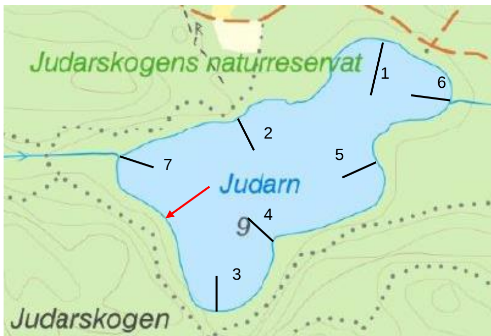
Figur 8 och 9. Ungefärliga lägen och sträckningar för transekter som inventerades i Judarn 2014. Röd pil markerar läge för vattenståndsinmätning. Kransslinga (på krattan) var en karaktärsart för sjön.
